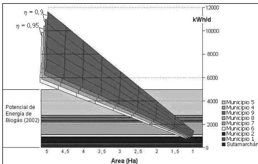
Figura 3 Necesidades de energía según el área de cultivo (ha) y producción potencial de biogas.
